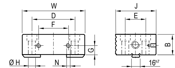
Art. 805O Ganascia fissa con gradino piccolo e grande Fixed jaw with small and large step
