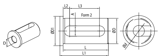
Bloccaggio con asola / Clamping with and slot
