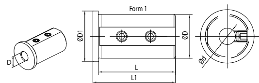
Bloccaggio con asola / Clamping with and slot
